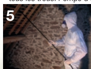
Pulvérisation du produit de traitement de bois D'XYL éco.R sur l'intégralité de la charpente
